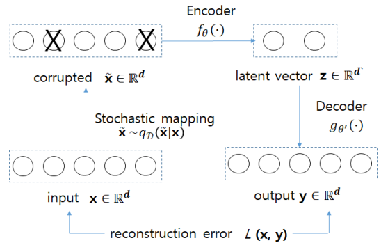
Fig. 2. Denoising AutoEncoder
